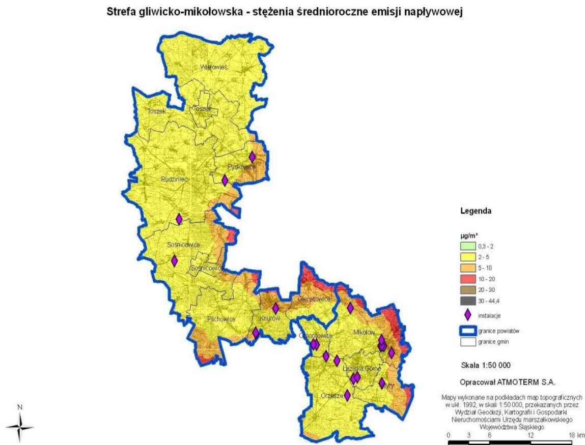
Rysunek 3.33. Rozkład stężeń średniorocznych pyłu zawieszonego PM10 spoza strefy gliwicko-mikolowskiej - prognoza 2020
