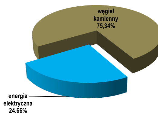
Struktura i wielkość emisji CO 2 [MgCO 2 /a]
