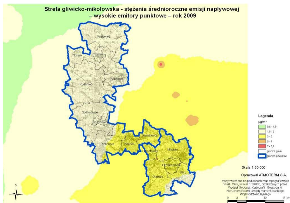
Rysunek 3.32. Stężenia średnioroczne emisji napływowej
