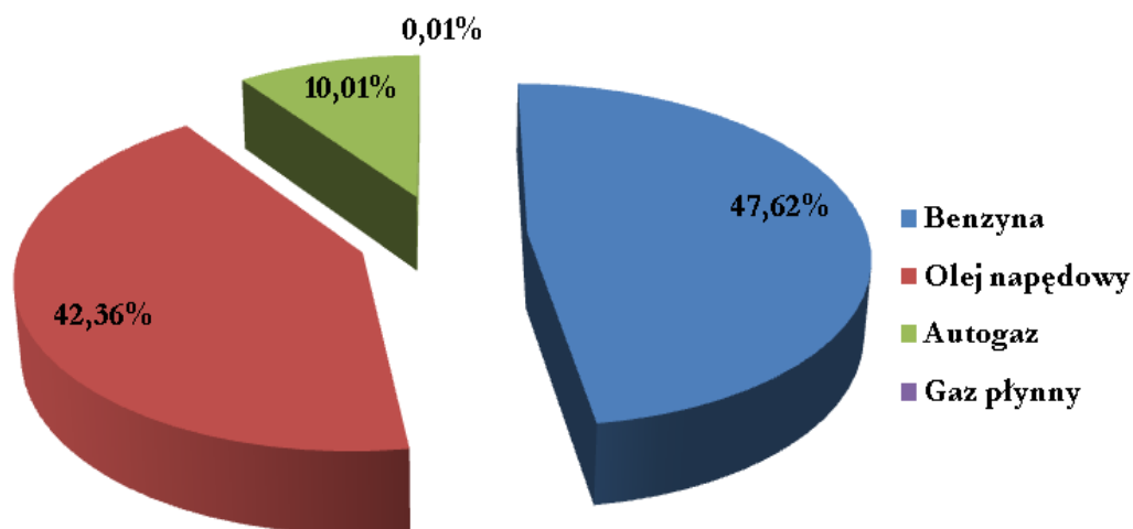
Rysunek 4.15. Struktura udziału poszczególnych paliw w emisji CO 2 przez transport
