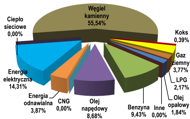
Struktura emisji CO 2 (MgCO 2 )
