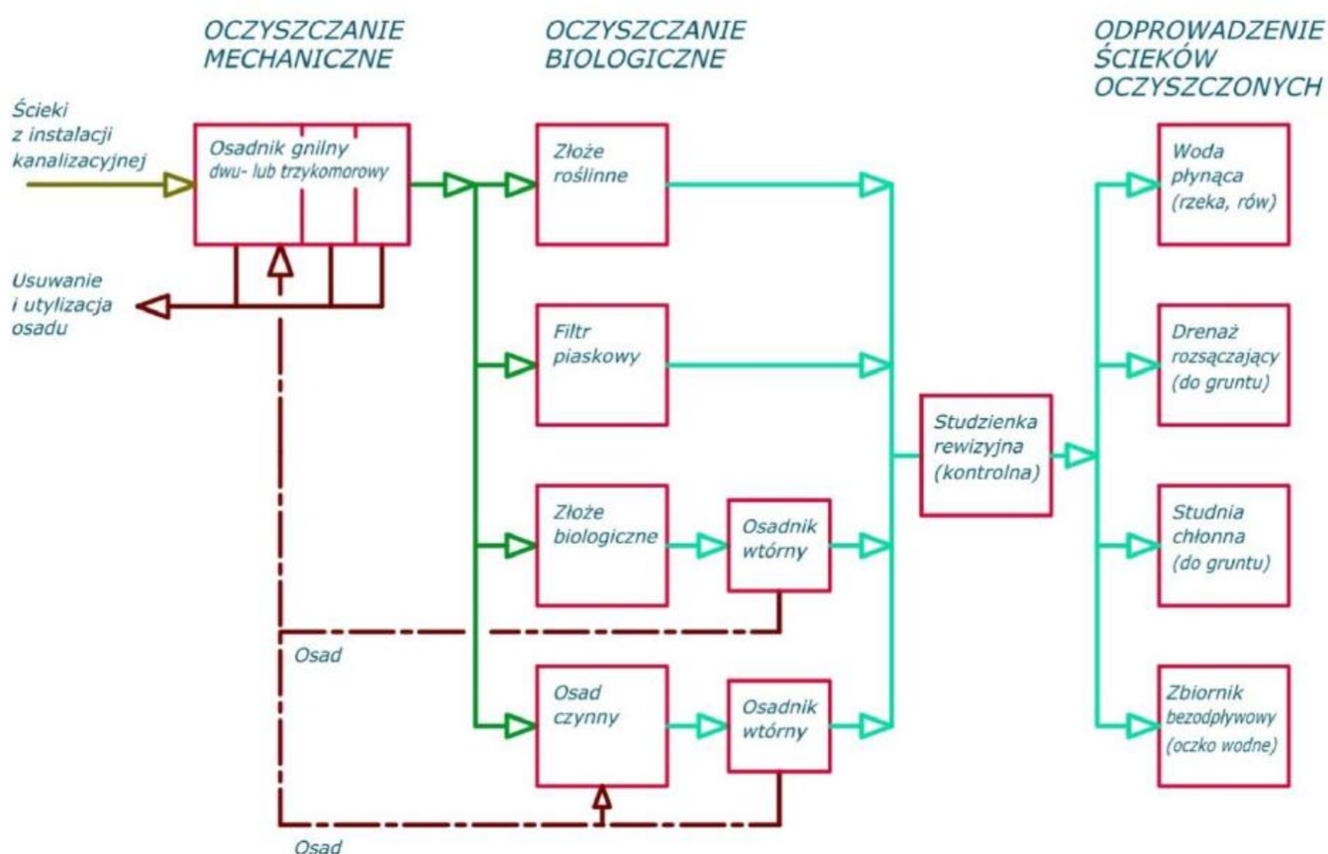
Rys.6. Schematy oczyszczania ścieków bytowych.
