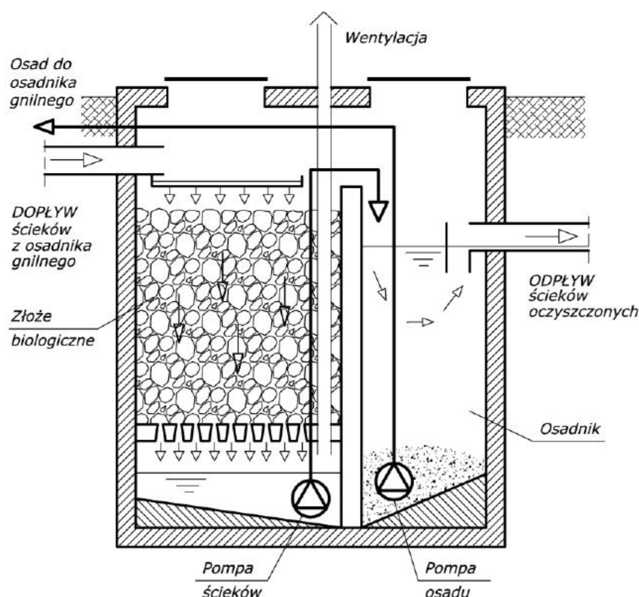
Rys. 7. Schemat oczyszczalni opartej na technologii złoż biologicznego.
