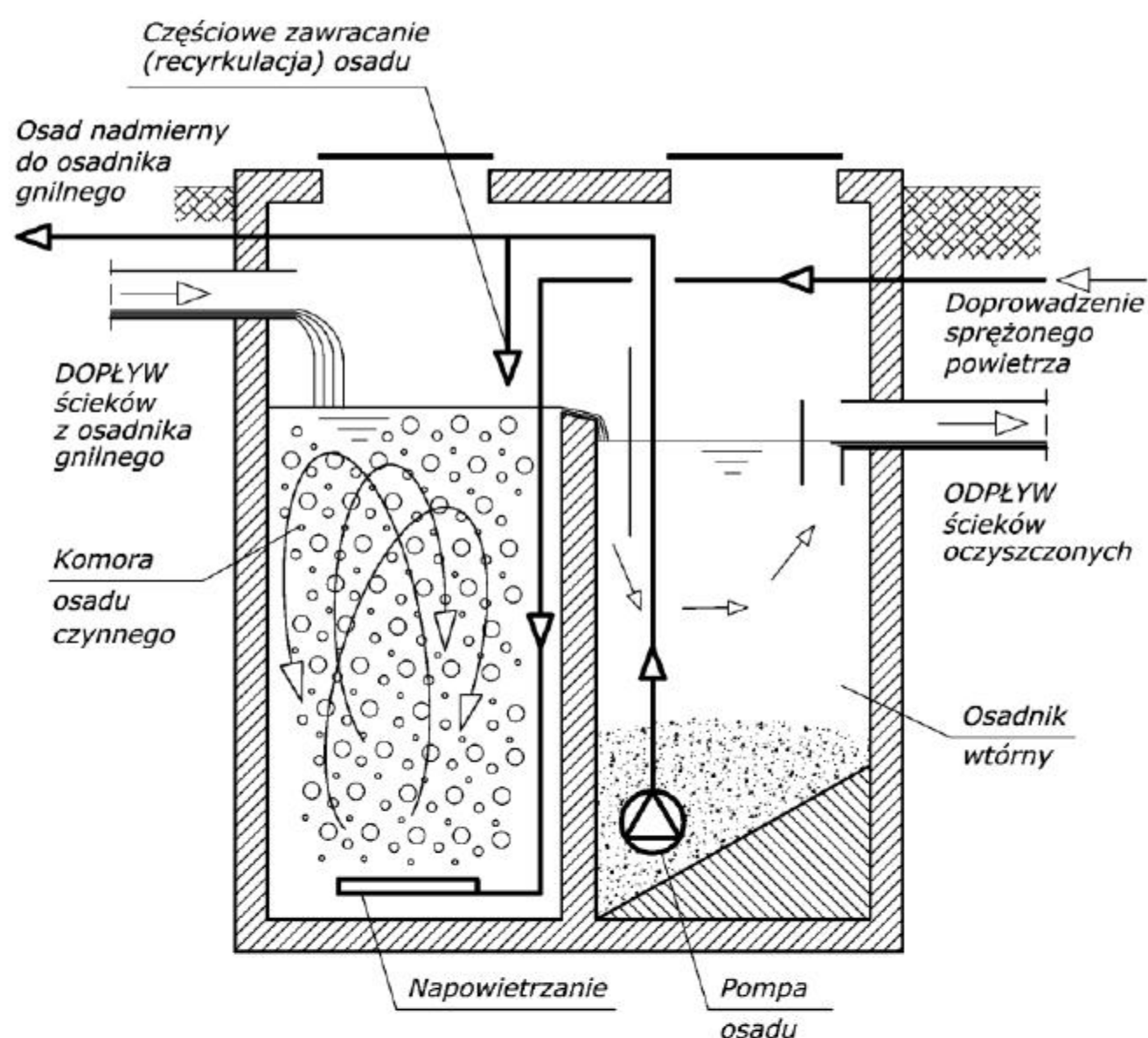
Rys. 8. Schemat oczyszczalni opartej na technologii osadu czynnego
