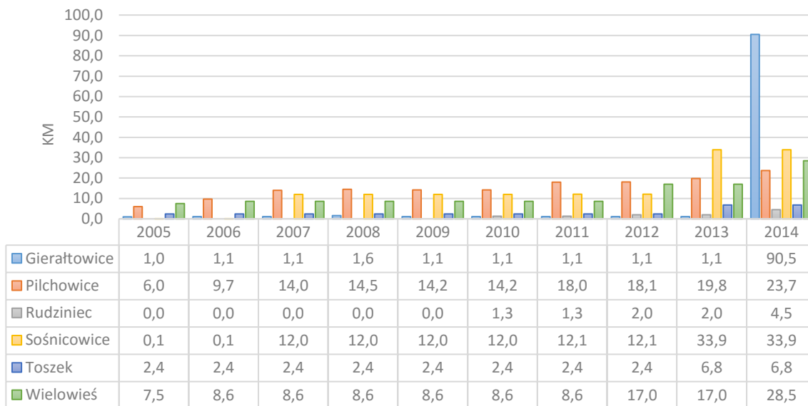
Wykres 93. Długość czynnej sieci kanalizacyjnej na obszarach wiejskich powiatu gliwickiego w latach 2005-2014
